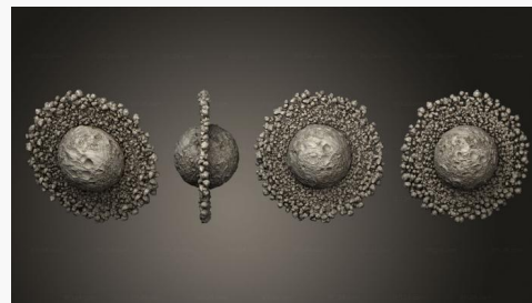
Экзопланета кольцевая луна 03
