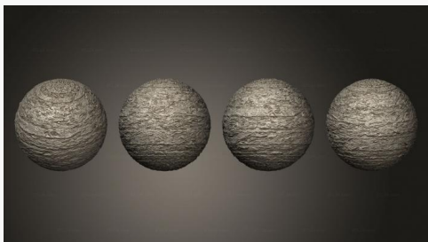
Экзопланета газовый гигант 01
