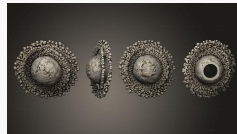
Экзопланета кольцевая planetthicc 02 SHPGM 1144 1800₽ →
