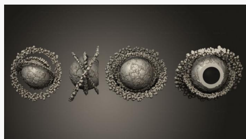
Экзопланета с кольцом 10
