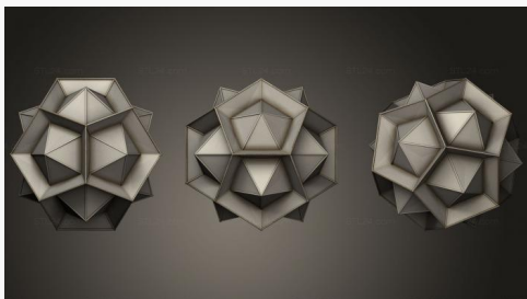
Додекаэдр Звездчатый тип 1
