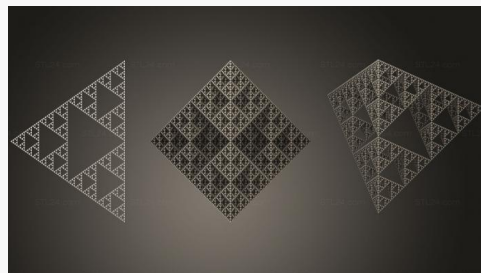
Четырехгранная прокладка уровень 6 SHPGM 0811 1800₽ →
