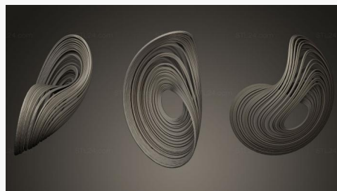
Странный аттрактор Хэдли 4
