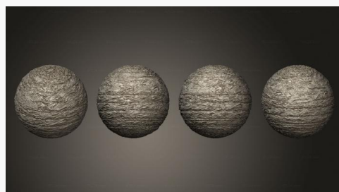
Экзопланета газовый гигант 06
