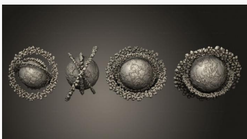
Экзопланета окольцованная планета 09
