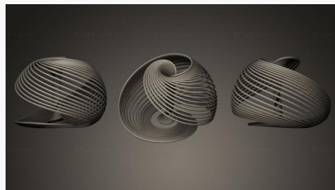
Странный аттрактор Аидзава 2 SHPGM 0108 1900₽ →
