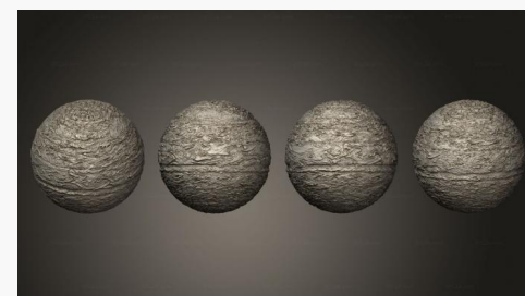
Газовый гигант экзопланеты 05
