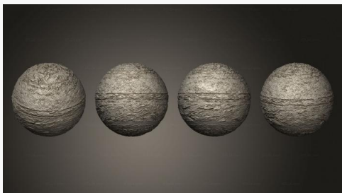
Газовый гигант экзопланеты 14
