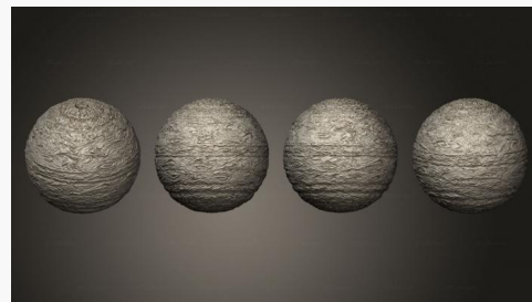
Экзопланета газовый гигант 02
