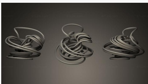
Странный аттрактор Хэдли 1 SHPGM 0111 1900₽ →
