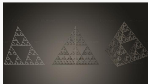
Четырехгранная прокладка уровень 7
