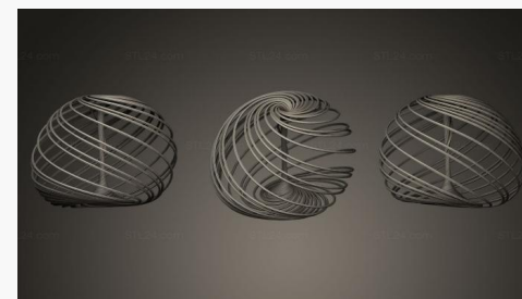
Странный аттрактор Аидзава 3 SHPGM 0109 1900₽ →
