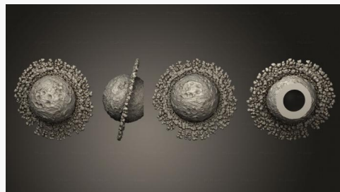
Экзопланета кольцевая луна 06
