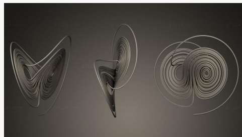
Странный аттрактор Лоренца 1 SHPGM 0114 1900₽ →
