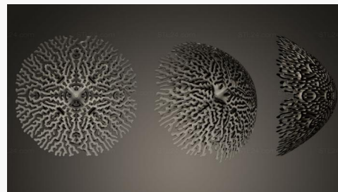
Серый Скотт с деформацией плоскости Среза SHPGM 0034 1900₽ →
