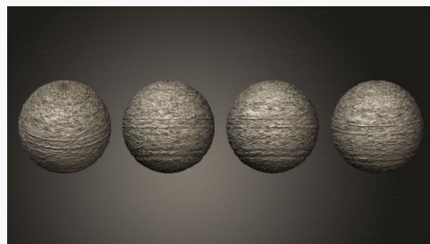
Газовый гигант экзопланеты 08
