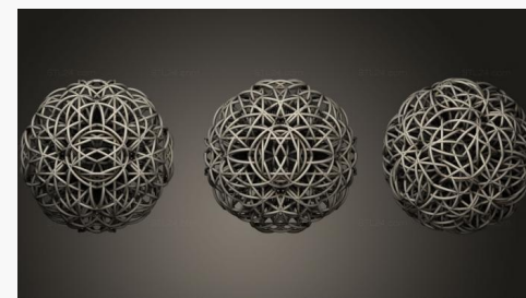
Темная материя завершена
