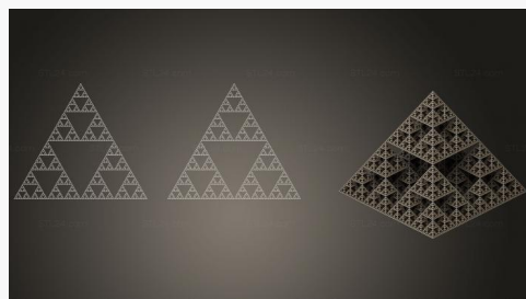
Прокладка Серпинского этап 7 SHPGM 0788 1800₽ →
