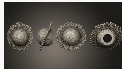
Экзопланета кольцевая луна 08
