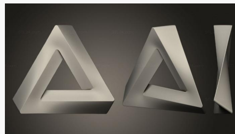
Треугольник Пенроуза SHPGM 0887 1900₽ →
