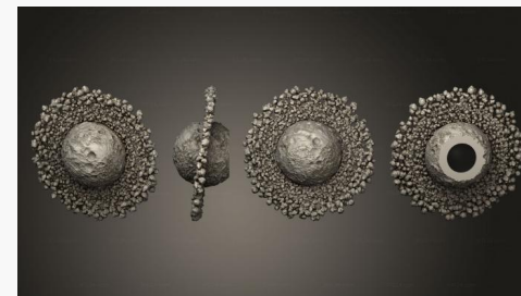
Экзопланета кольцевая луна 04
