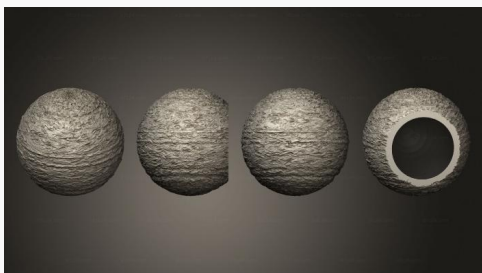
Экзопланета газовый гигант 08 поля
